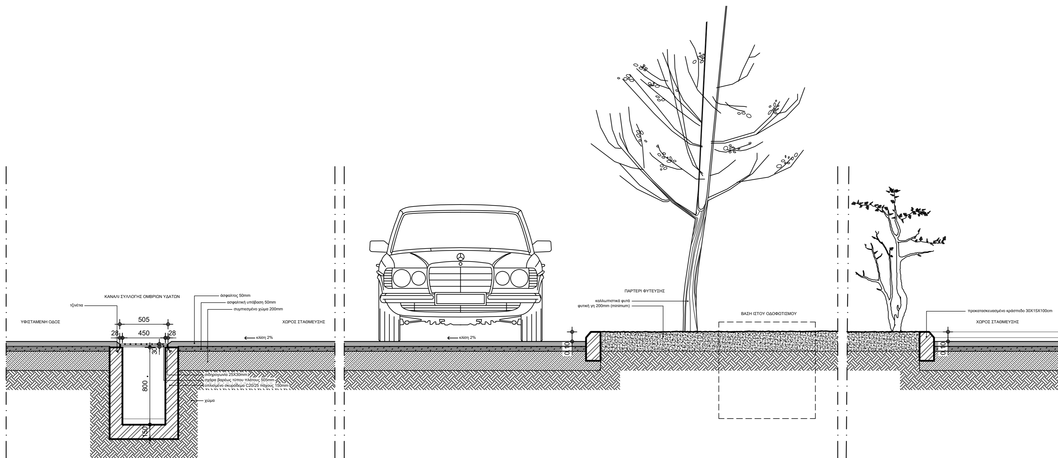
ΤΥΠΙΚΗ ΚΑΤΑΣΚΕΥΑΣΤΙΚΗ ΛΕΠΤΟΜΕΡΕΙΑ ΧΩΡΟΥ ΣΤΑΘΜΕΥΣΗΣ 1:10
